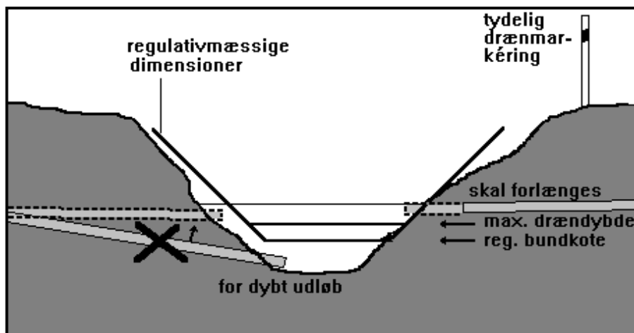
Forkert og korrekt anlagt drænudløb.
